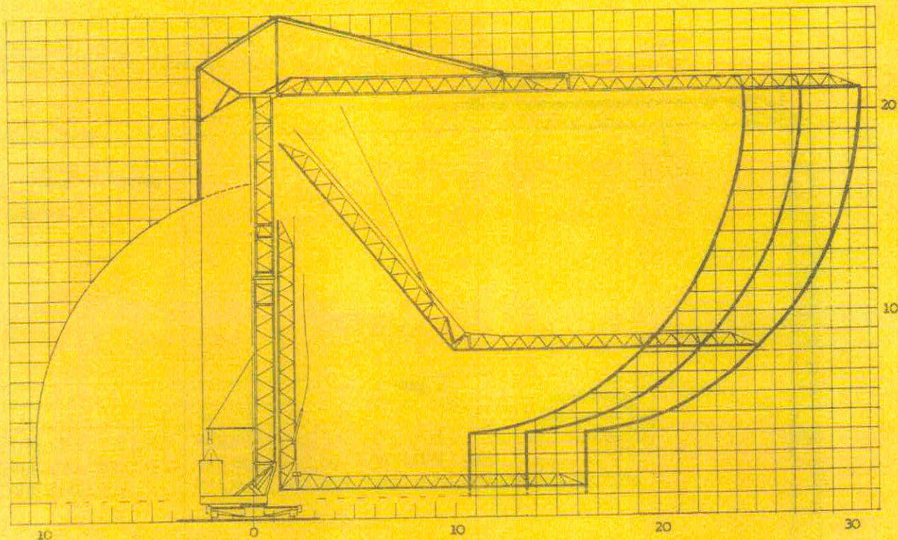
AUTOCALAGE DE LA GRUE AUTOMATISCHES AUFGLEISEN AUTOWEDGING OF THE CRANE
