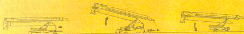
AUTOCALAGE DE LA GRUE AUTOMATISCHES AUFGLEISEN AUTOWEDGING OF THE CRANE
